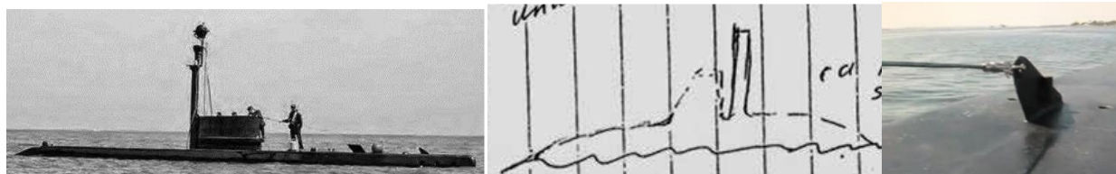
Italiensk COSMOS 506-SX (23 meter) i Colombia og en tegning av Type 2-ubåt (20-25 meter) i Stockholms sydlige skjærgård 1987. Begge har en høy snorkelmast bak tårnet. Til høyre: vaier (festet i baugen) som går til tårnets topp.
