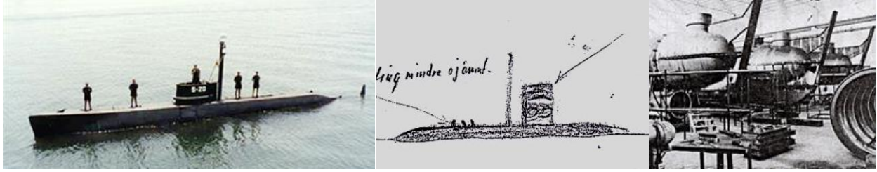
Italienskygget COSMOS SX-506 (23 meter) og en tegning av en Type 2-ubåt med den samme størrelsen (20-25 meter) fra oktober 1982 under ubåtsjakten i Hårsfjärden. Begge ubåtene har en høy snorkelmast bak tårnet. Til høyre: masseproduksjon av COSMOS SX-506 i Livorno i begynnelsen av 70-tallet.
